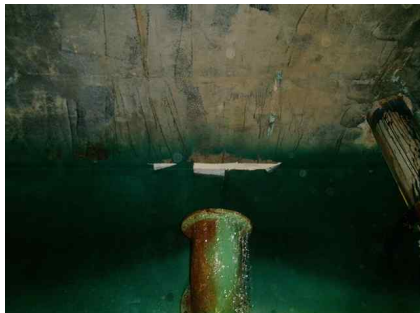
<배수지 1지 상부슬래브 도장손상>
